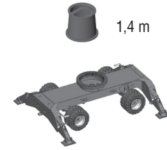
XL-undercarriage XL-Unterwagen
